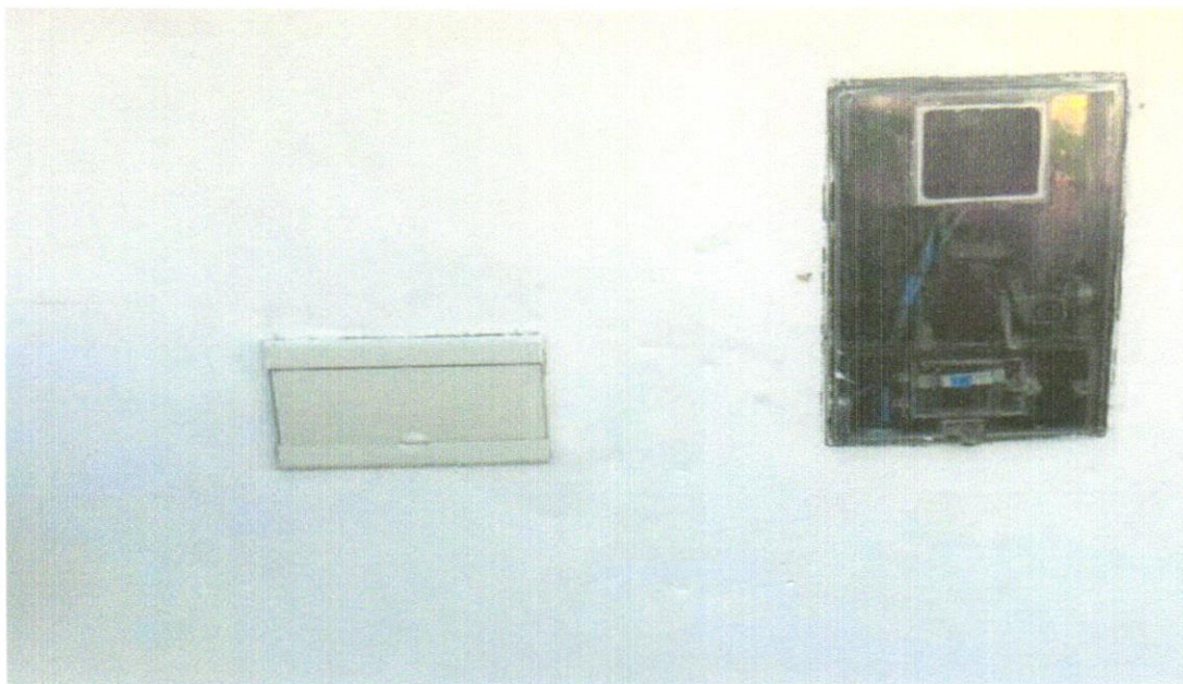
Foto 11 - CAIXA DE MEDIÇÃO DIRETA ATÉ 200A CONFECCIONADA EM CHAPA GALVANIZADA E PINTADA ELETROSTÁTICAMENTE D=100X60X15 CM e QUADRO DE DISTRIBUIÇÃO DE ENERGIA EM PVC, DE EMBUTIR, SEM BARRAMENTO, PARA 6 DISJUNTORES - FORNECIMENTO E INSTALAÇÃO. AF_10/2020
